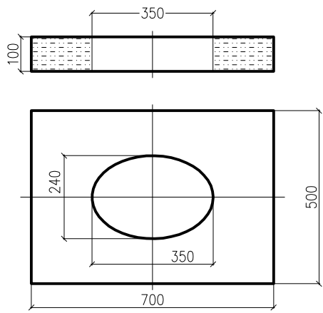
Płyta hydrantowa góra 2
