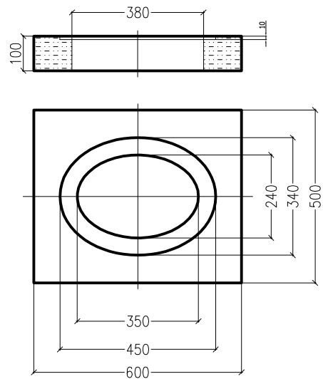
Płyta hydrantowa dół
