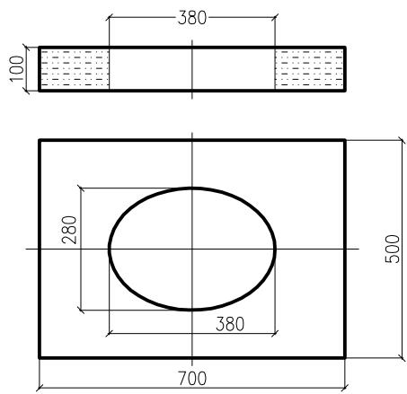
Płyta hydrantowa góra 1
